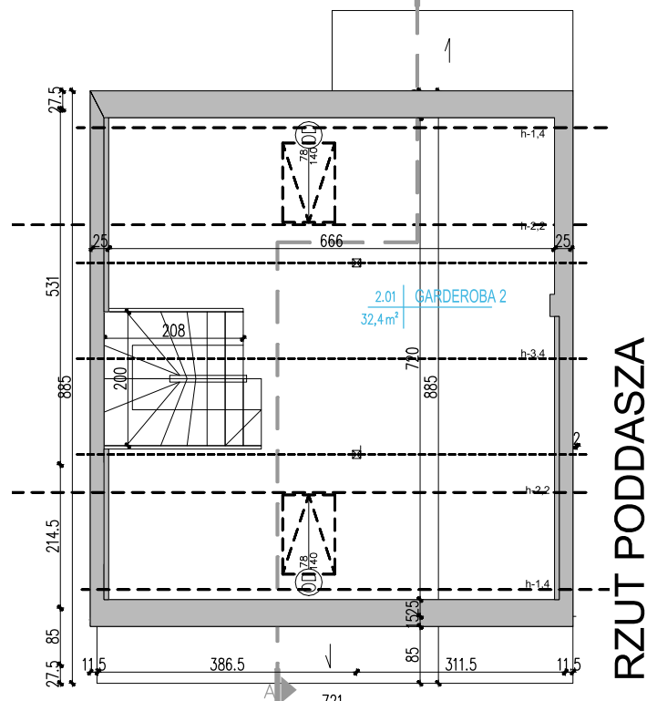
RZUT PIĘTRA
