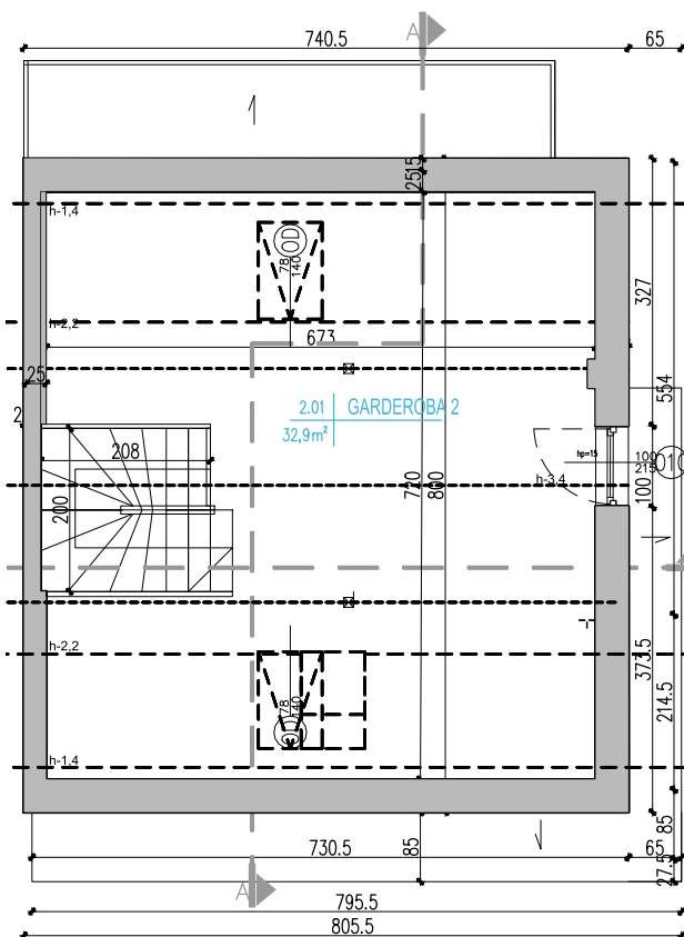
RZUT PIĘTRA
