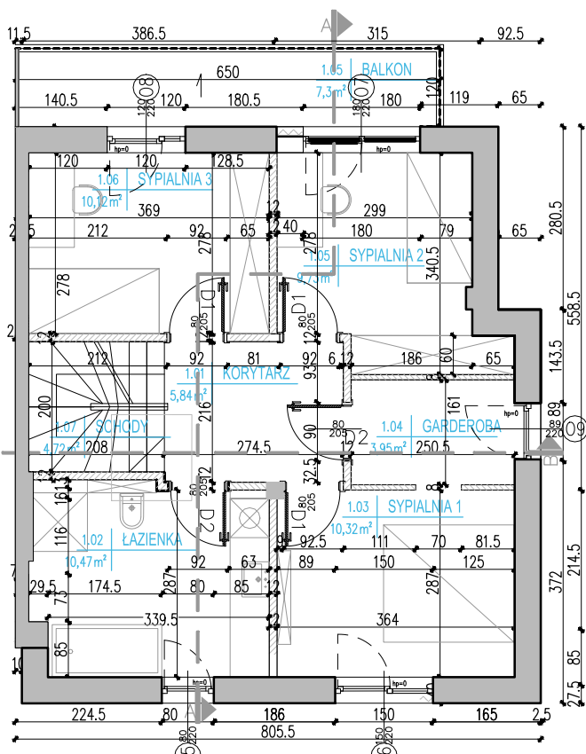
RZUT PIĘTRA
