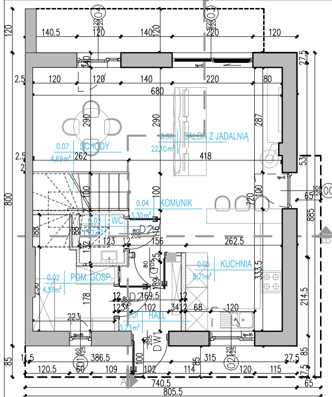
RZUT PARTERU
