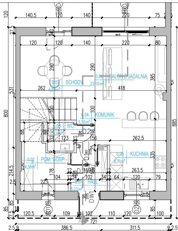
RZUT PARTERU
