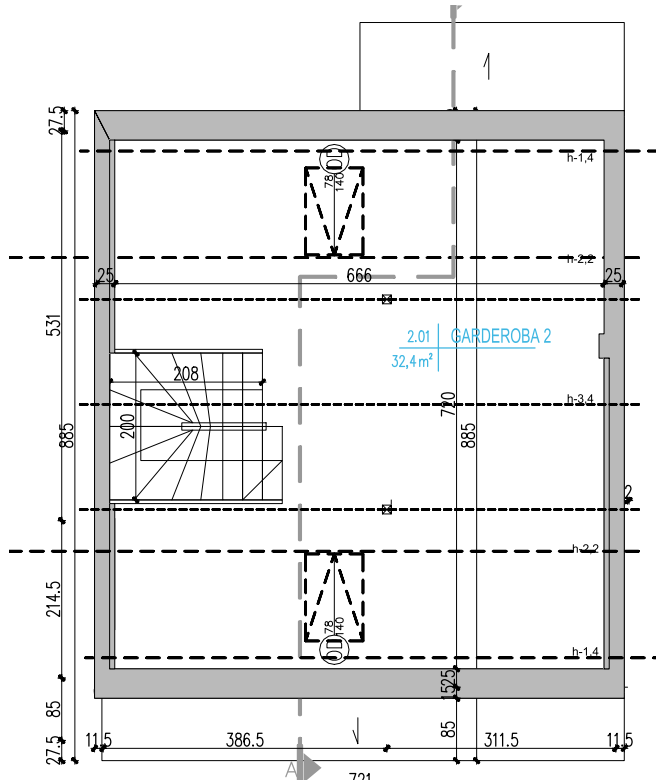
RZUT PODDASZA
