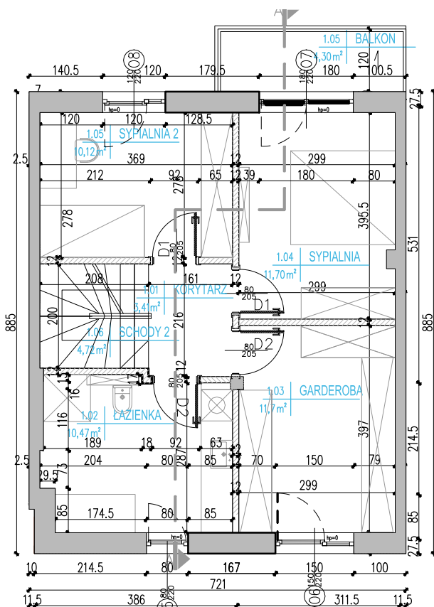
RZUT PIĘTRA
